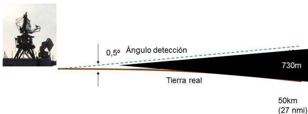
Figura 1: Cono de sombra de un RADAR hasta los 50km.
