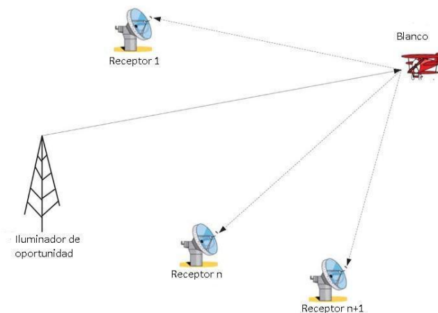
Figura 3: RADAR Multiestático
